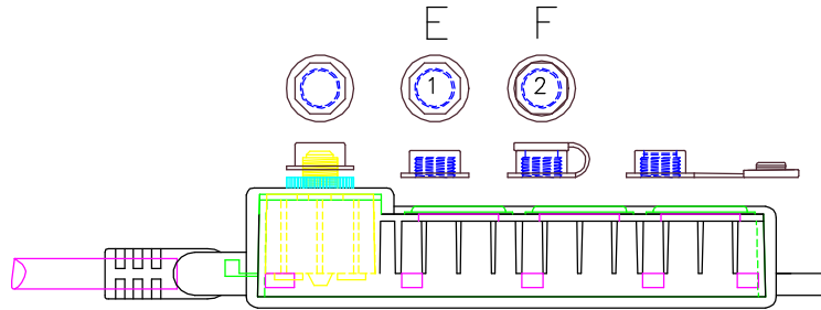
外模上視圖
