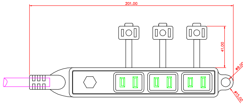
外模上視圖
